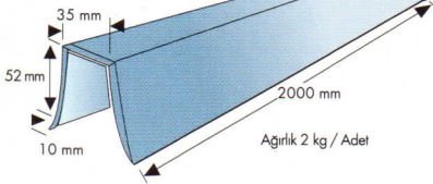
Köseli Sırt Mahya
