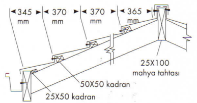
Decra ve Corona için Kadran Aralıkları
